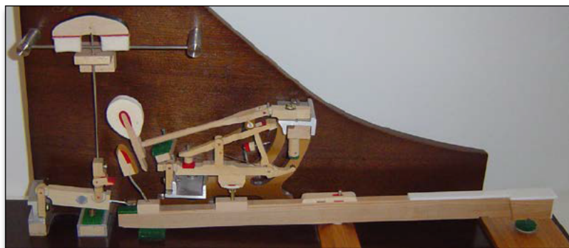
Mécanique à marteaux d'un piano à queue
